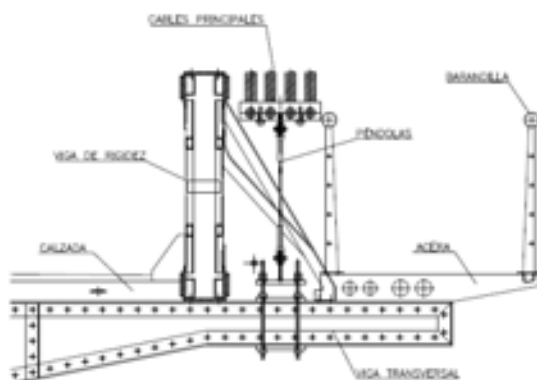
Fig 23: Sección transversal de puente rehabilitado
