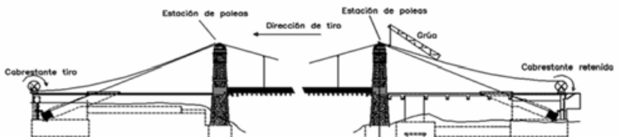
Fig. 8: Esquema de proceso de retirada de cable principal
