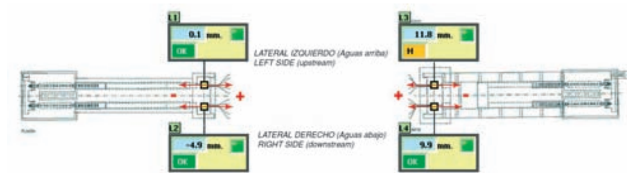
Figura 42. Sistema de instrumentación. Gráfico de control. Figure 42. Instrumentation system. Monitoring graph.
