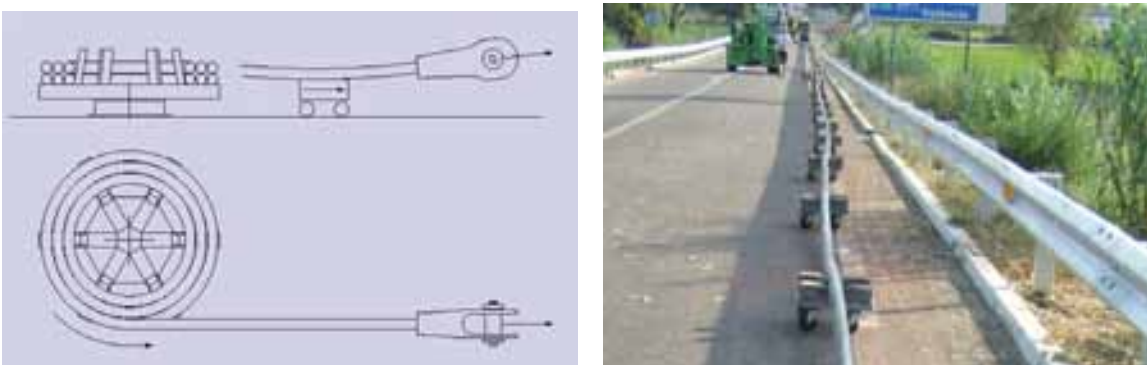
Fig. 14: Tendido sobre el suelo del cable principal nuevo
