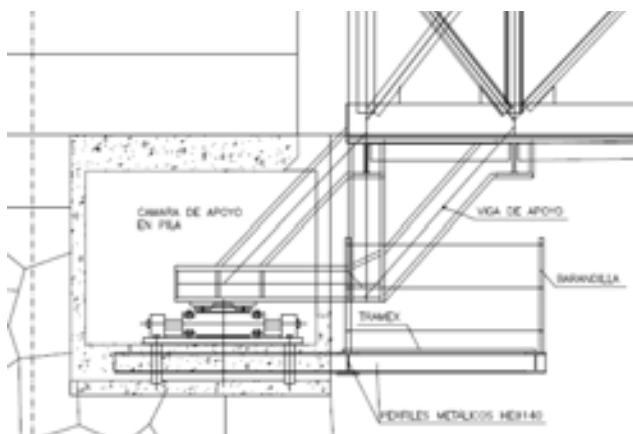
Fig 22: Detalle nuevas cámara de apoyos y apéndices metálicos
