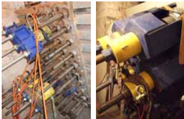
Fig. 17: Equipos de tesado sobre los cables principales (antiguos y nuevos) en emparrillados de anclaje
