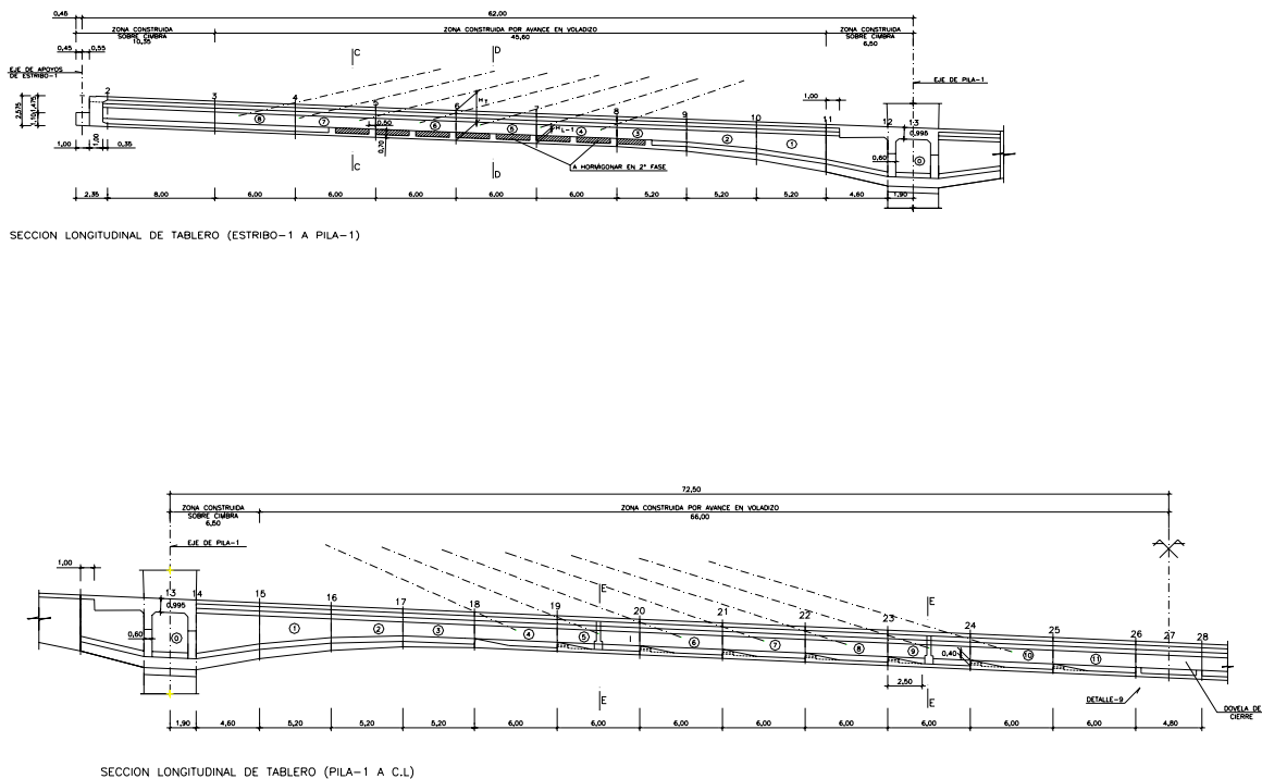
Fig. 3 Sección longitudinal del tablero
