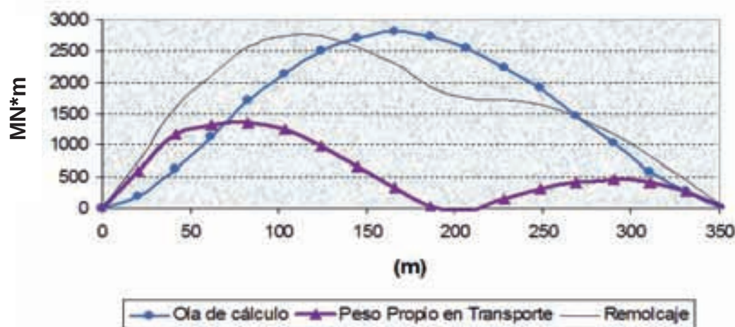
Figura 5.3.6. Momentos flectores longitudinales.
