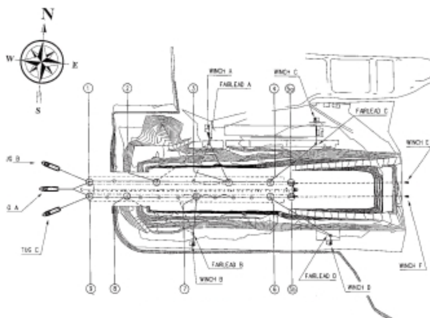
Figura 7.4.6. Secuencia de maniobras de salida de la dársena (Fase 3.)
