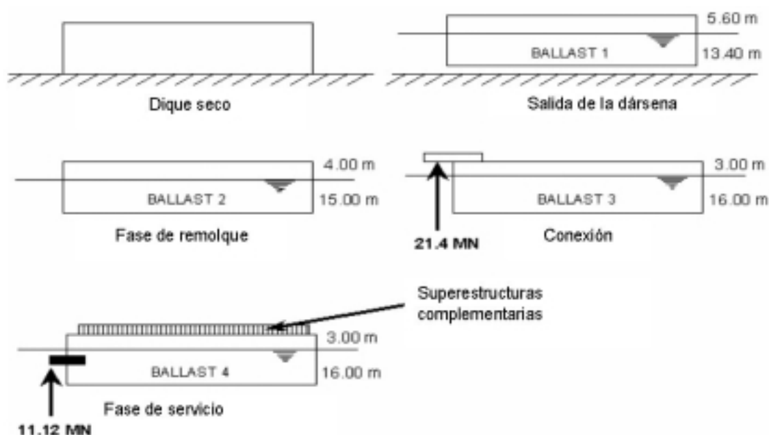
Figura 2.2.4. Operaciones marítimas.
