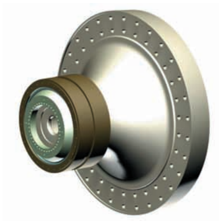
Figura 5.1.6 Perspectiva del eje troncocónico.
