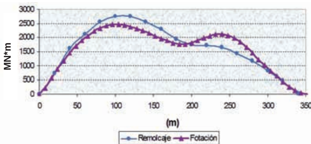
Figura 5.3.7. Comparación de momentos flectores longitudinales después de la flotación.
