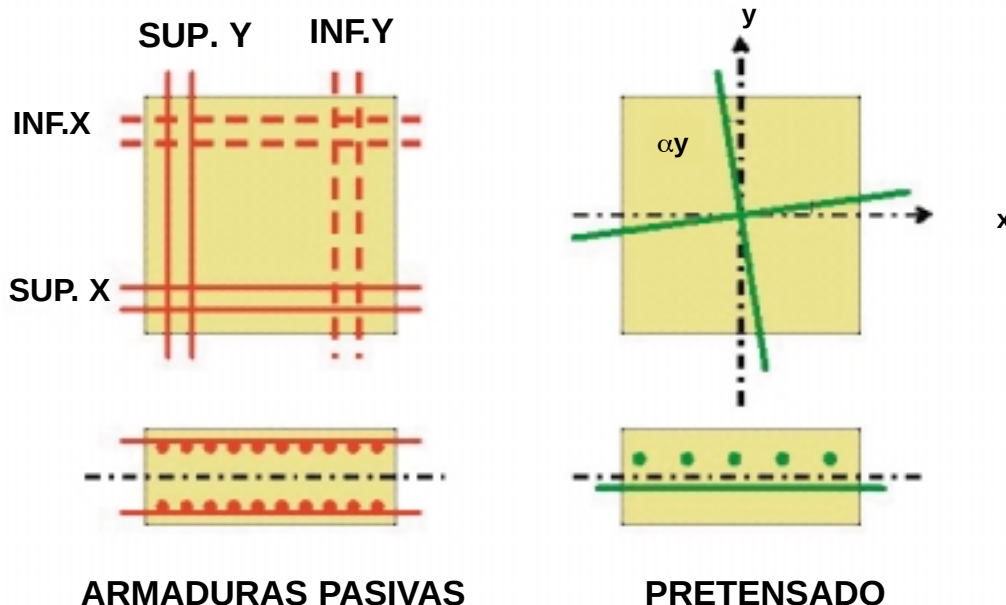
Figura 2.6.4. Armado ARMATEC.
