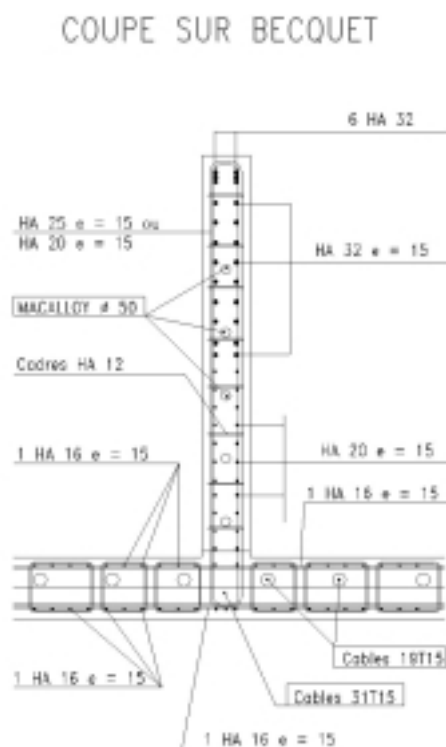
Figura 2.7.2. Sección de rigidizadores.
