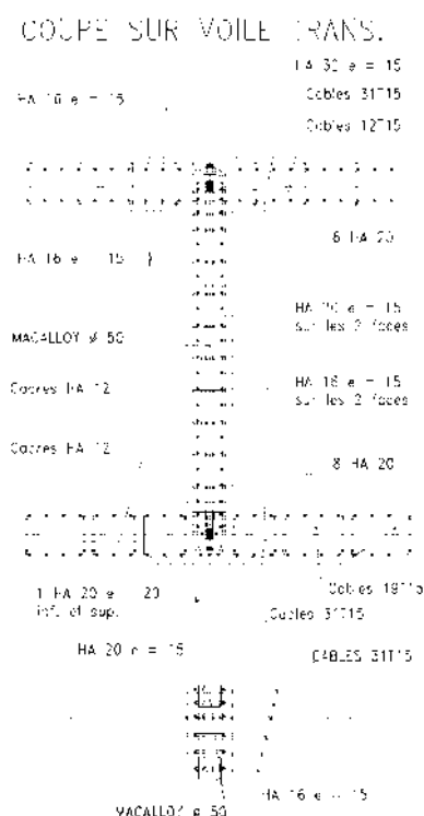
Figura 2.7.4. Sección de muro transversal.
