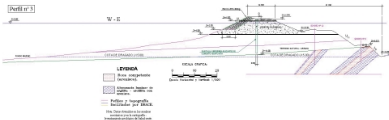
Figura 7.3.3. Perfil.
