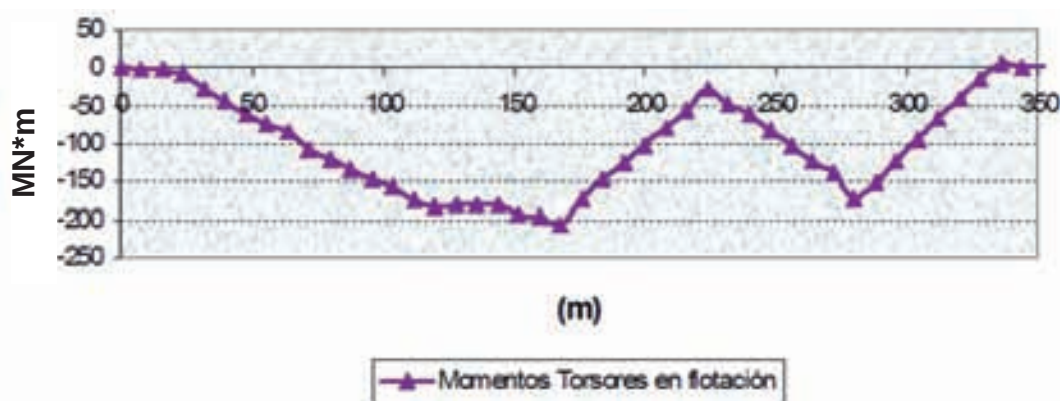
Figura 5.3.8. Momentos torsores en flotación.
