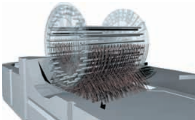
Figura 6.4.5. Fases de hormigonado de la rótula.
