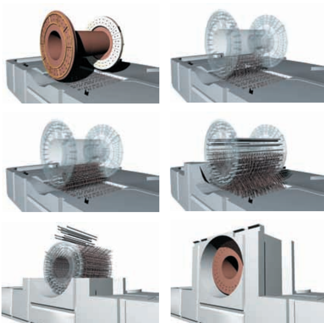
Figura 5.4.7. Modelización del armado de la rótula.
