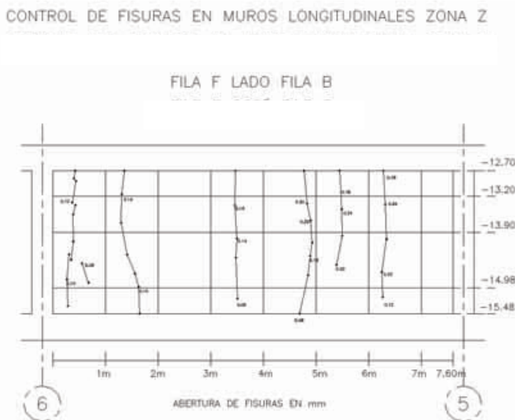
Figura 5.6.1. Mapa de fisuras obtenido en una de las primera observaciones.
