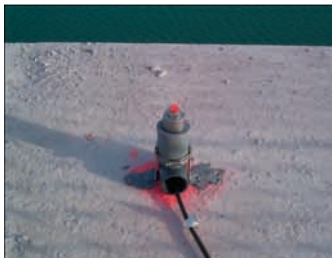
Figura 5.7.8. Sensores de presión hidrodinámica dispuestos en cubierta.
