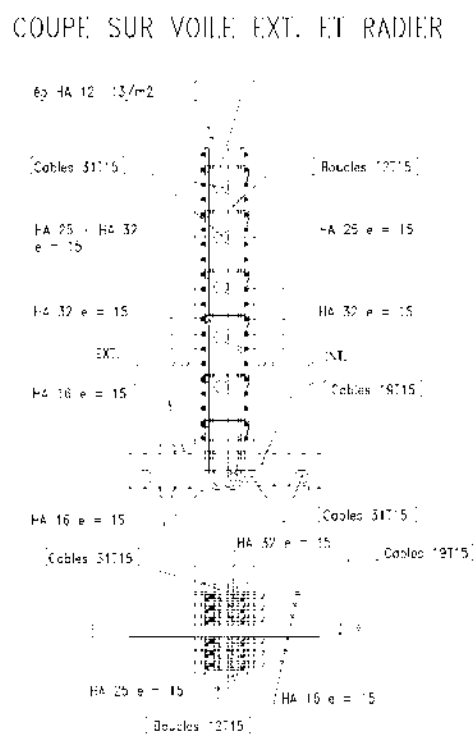
Figura 2.7.3. Sección de muro exterior y solera.
