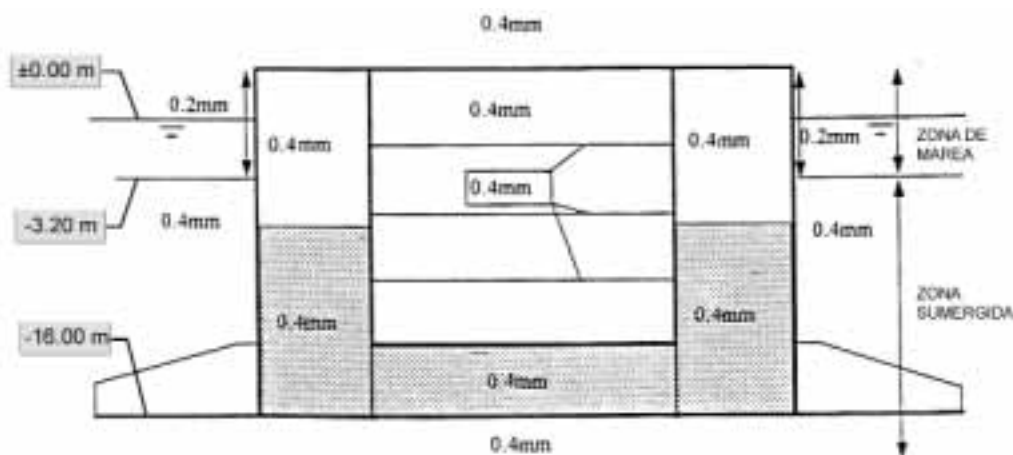
Figura 2.5.1. Limitación de abertura de fisura.
