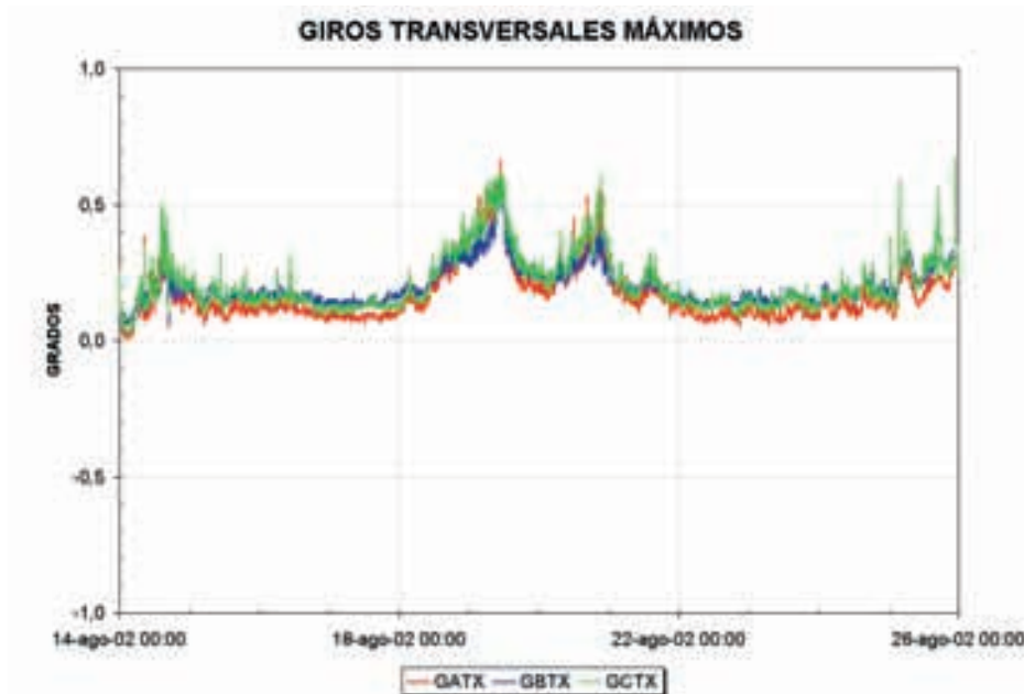
Figura 5.7.14. Giros transversales máximos cada 10´.
