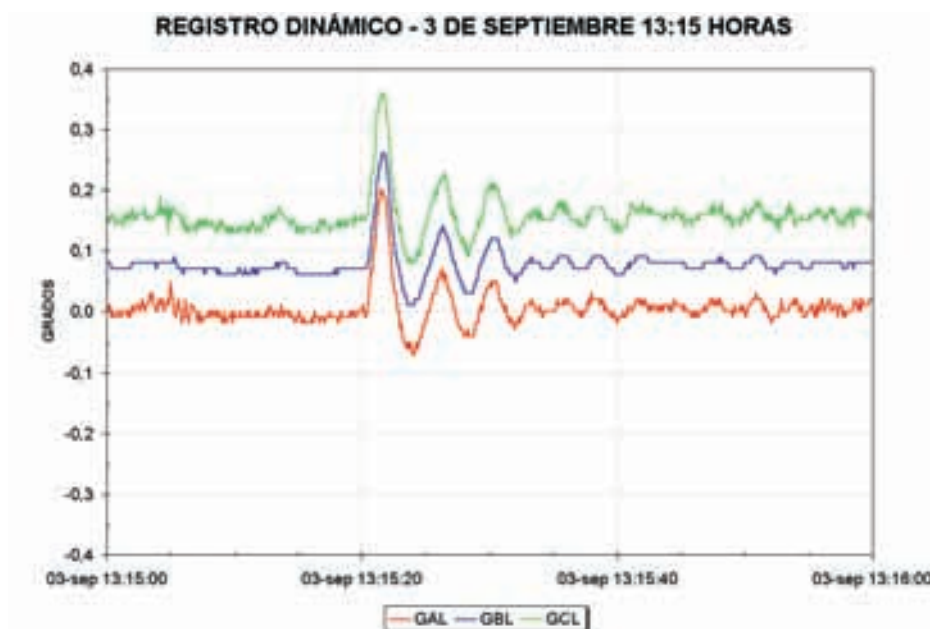
Figura 5.7.15 b). Giros longitudinales durante las operaciones de conexión de la rótula (3/09/02). Detalle del registro dinámico de los giros correspondientes al período de 10 minutos entre las 13.07 y las 13.17 horas.
