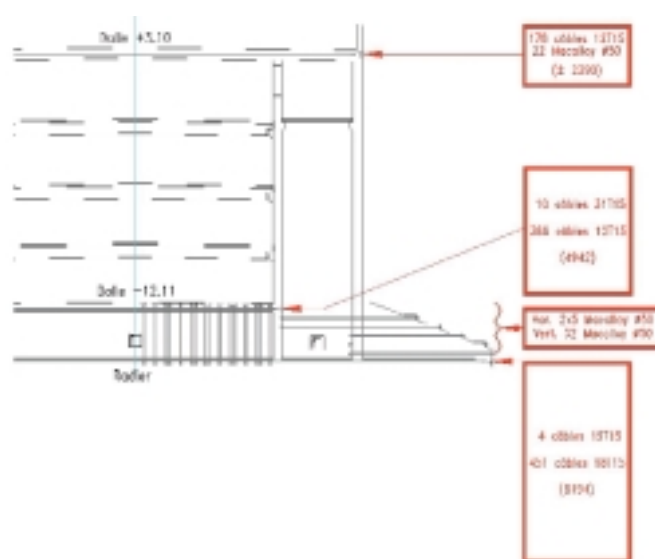
Figura 2.8.3. Pretensado transversal.
