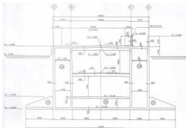
Ilustración 4 Sección transversal tipo.
