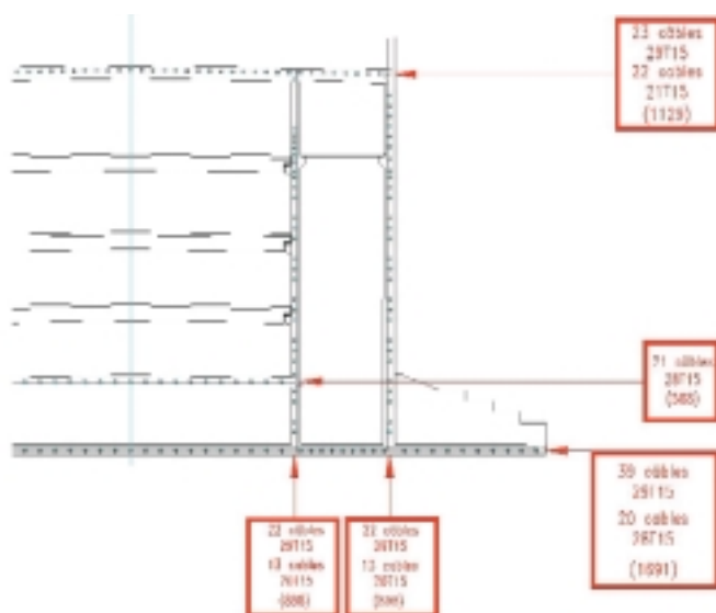
Figura 2.8.2. Pretensado longitudinal.
