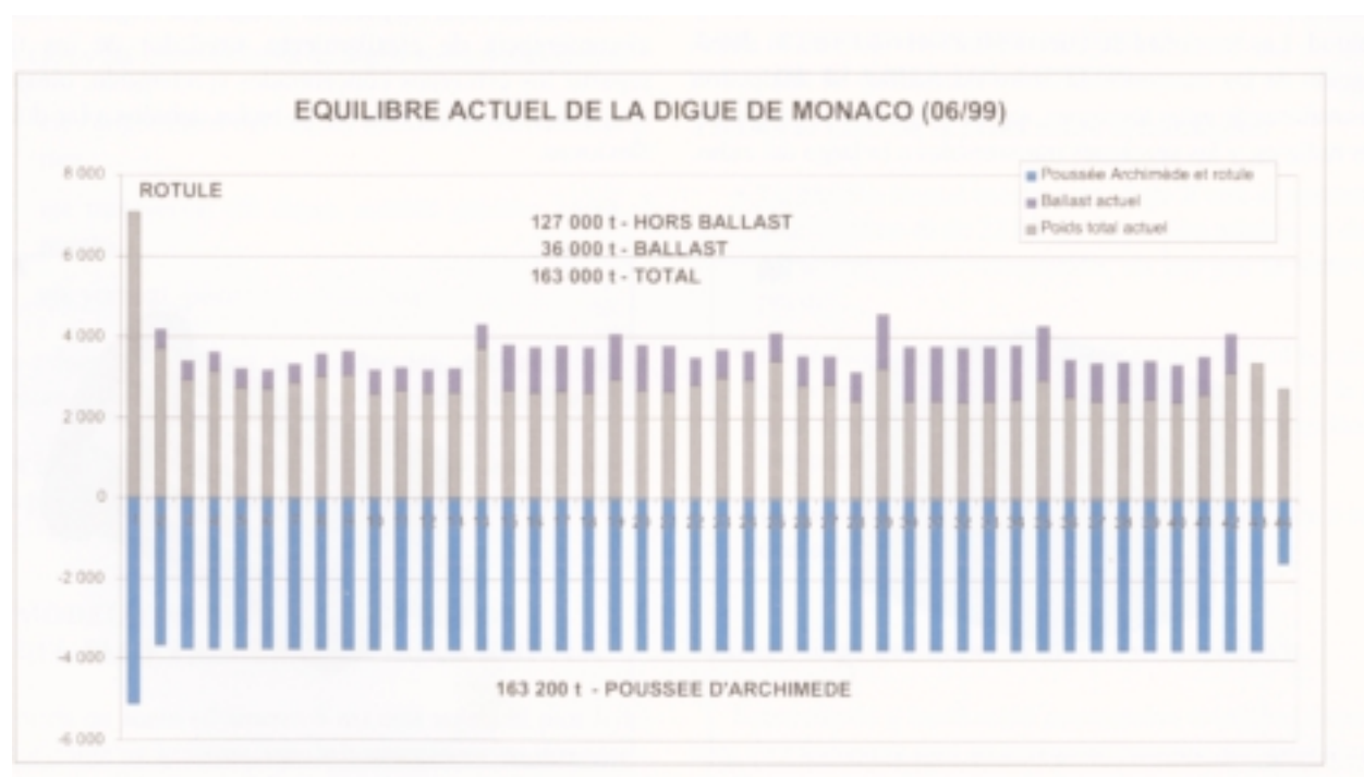
Figura 2.10.1. Fuerzas de equilibrio del dique.
