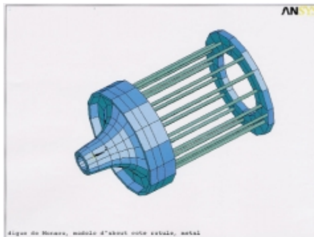
Figura 2.9.2. Elementos finitos de la rótula.
