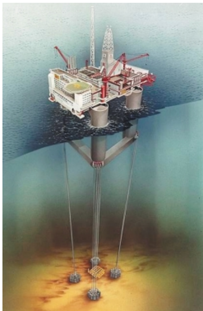
Figura 1.5. Heidrun T.L.P.
