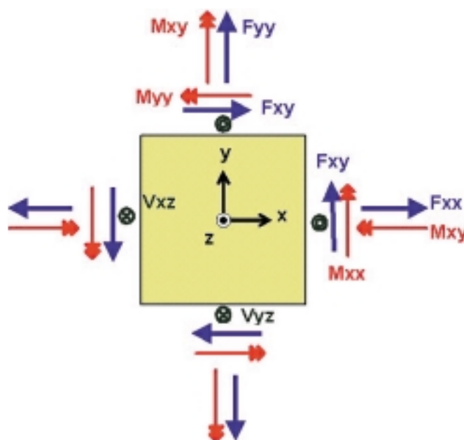
Figura 2.6.3. Esfuerzos ARMATEC.
