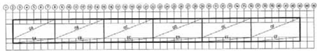
Figura 5.3.1. Distribución en planta de los tanques de lastrado.
