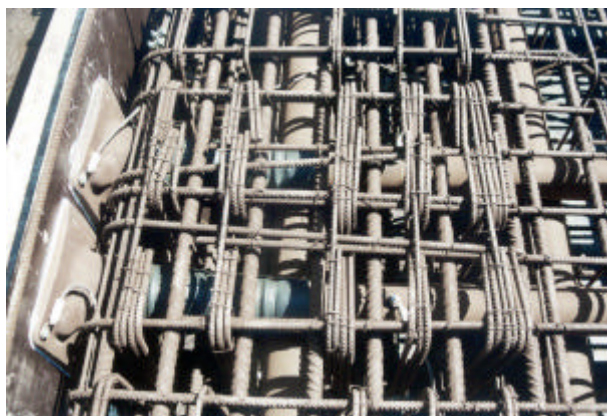
Ilustración 8 Anclajes BBR CONA Compact instalados.
