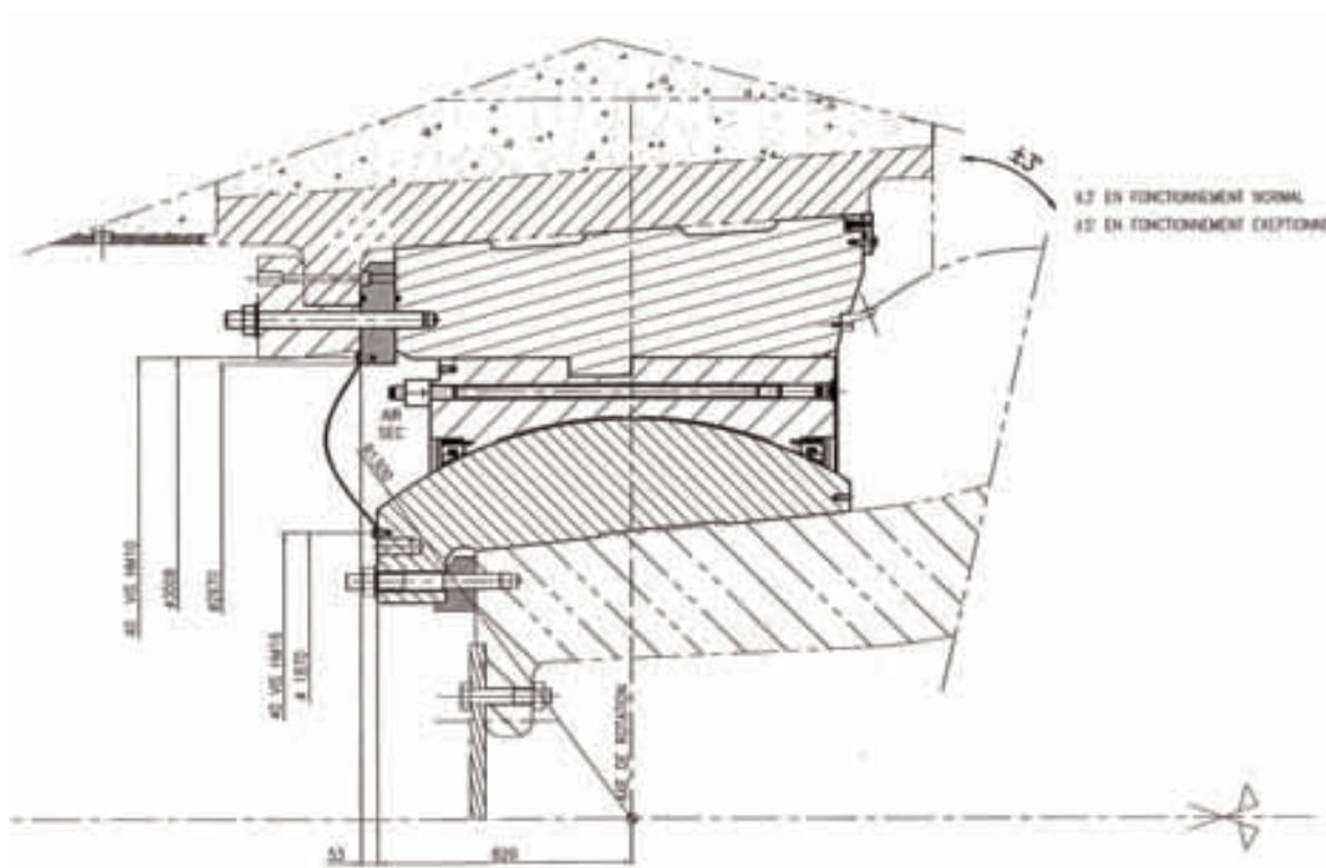
Figura 5.1.5. Conjunto rotula/casquillo/manguito.
