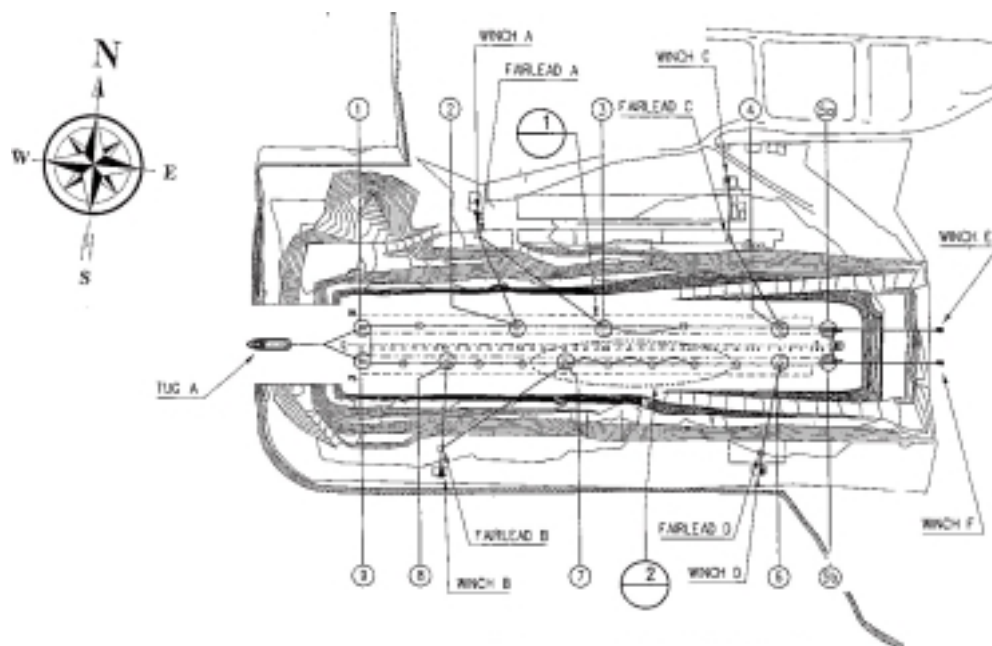
Figura 7.4.6. Secuencia de maniobras de salida de la dársena (Fase 1.)
