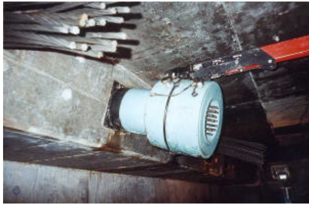
Ilustración 11 Tesado en el interior de las celdas estancas.
