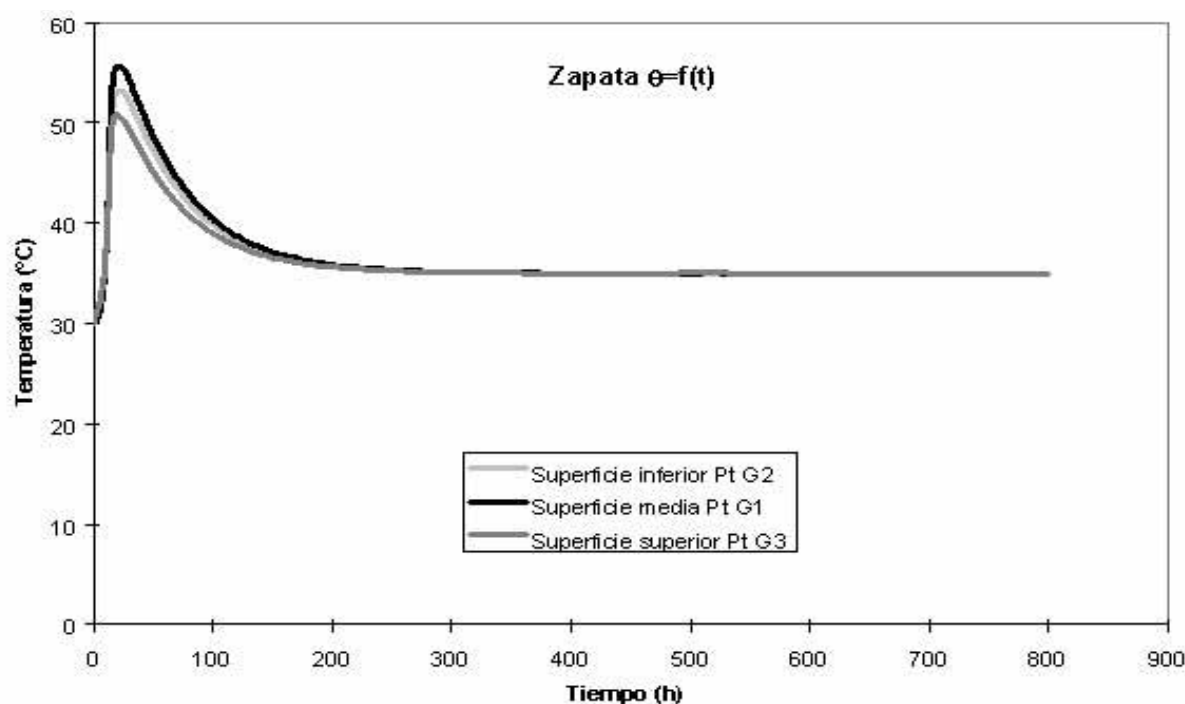
Figura 3.3.5. Temperaturas en verano en zapata con espesor tipo.
