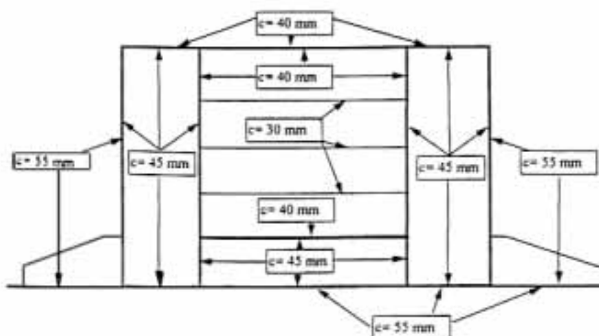
Figura 2.5.2. Recubrimientos.
