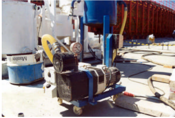
Ilustración 16 Bomba de vacío.
