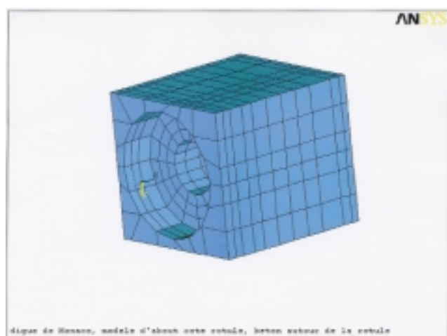
Figura 2.9.1. Elementos finitos del macizo de la rótula.
