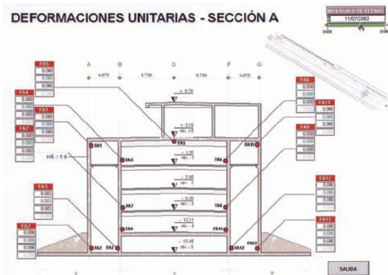
Figura 5.7.10b. Panel sinóptico de valores estadísticos de varios canales para un período de 10'.
