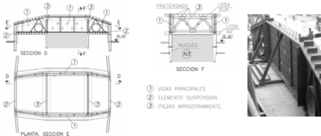
Figura 7. Estructura de suspensión en coronación de núcleo N3
