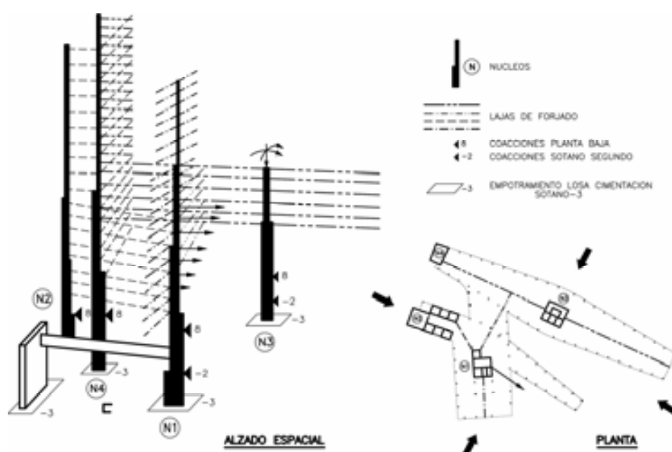
Figura 9. Esquema espacial global frente a acciones horizontales
