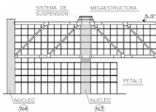
Figura 6. Edificio Portaaviones (Sección C fig. 2)
