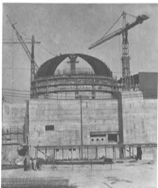
Fot. 11. Montaje de la cúpula metálica.
