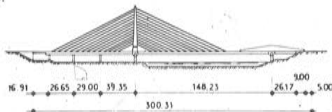
Figura 5.— Sección longitudinal del puente de HOECHST.
