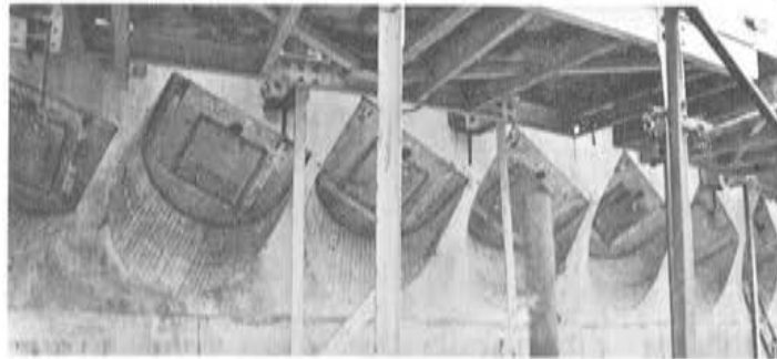
Fot. 17. Los cajetines para los anclajes de los tendones de la cúpula.
