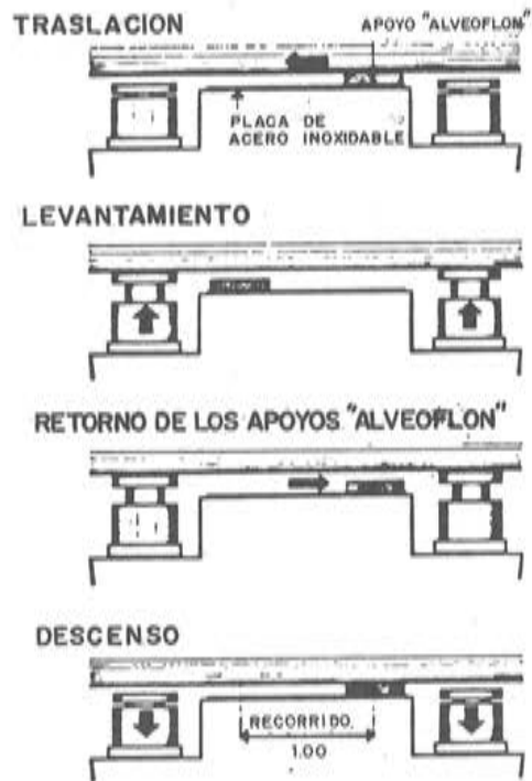
Fig. 24. Apoysos deslizantes en Acueducto de Abeou.
