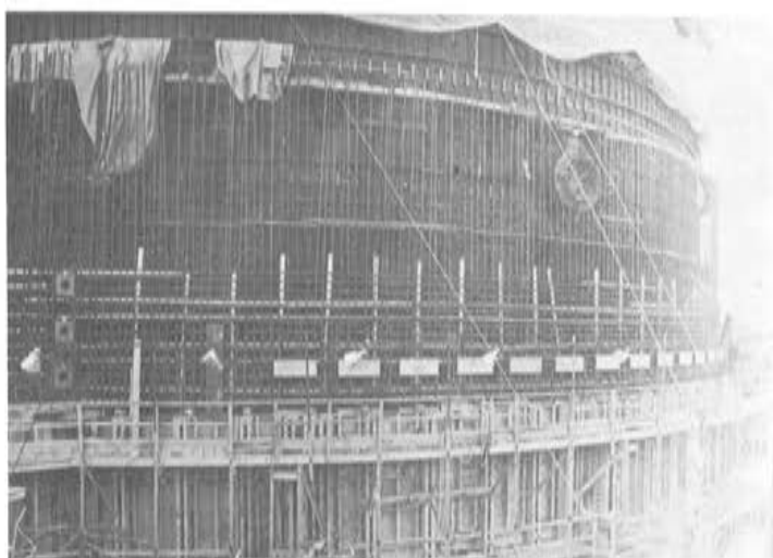
Fot. 6. Vista general del muro en construcción del edificio de contención. Puede verse el encofrado trepante, la colocación de vainas verticales y horizontales, y la armadura.
