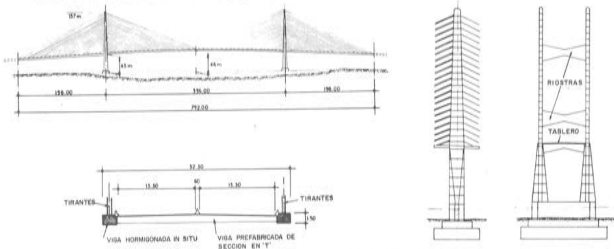
Figura 22.— Proyecto del puente de DAME POINT.
