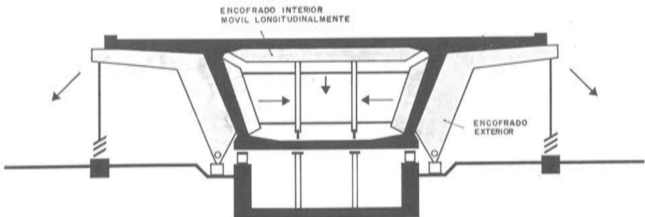
Fig. 21. Encofrados internos en Loisach.
