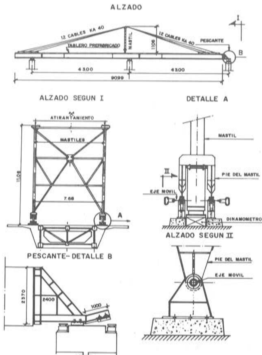
Fig. 16. Viaducto sobre el Boivre. Atirantamiento.
