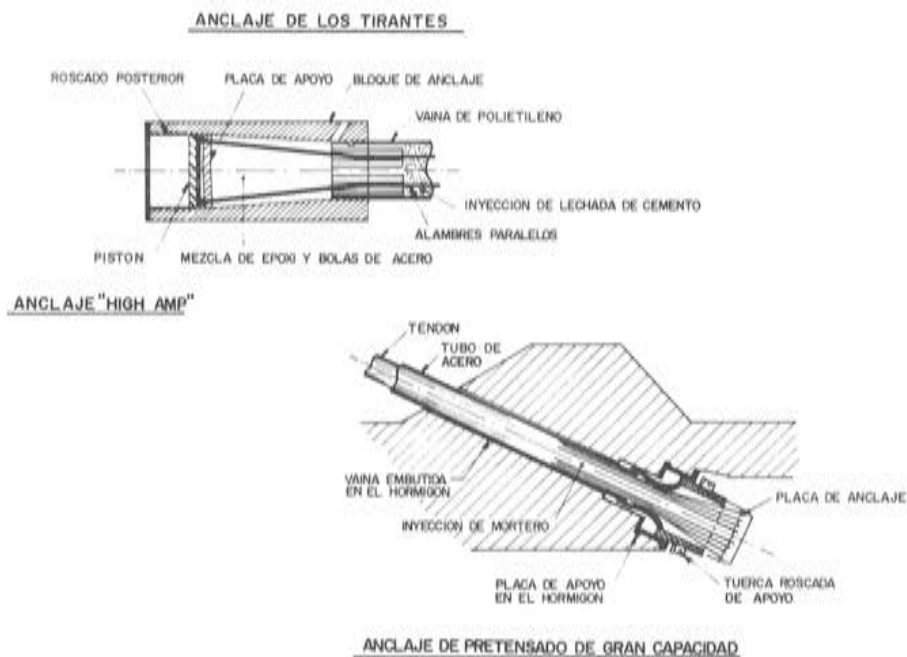
Figura 3.— Anclaje de los tirantes.
