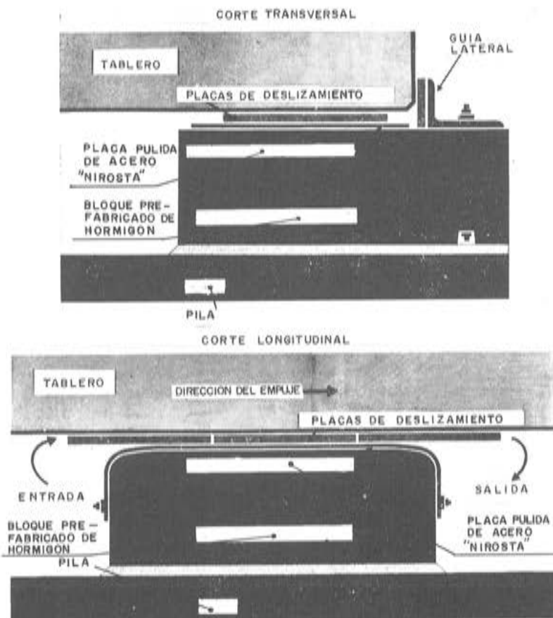
Fig. 25. Apoysos deslizantes del puente de Loisach.
