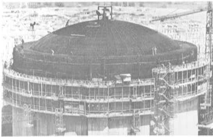
Fot. 13. Armadura del Anillo de borde de la cúpula e inicio de la armadura interior de la cúpula.
