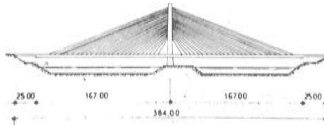
Figura 7.— Sección longitudinal del puente de OTTMARSHEIM.
