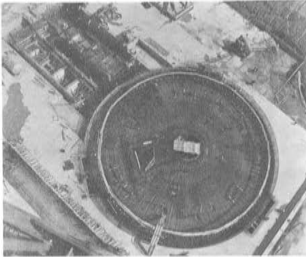
Fot. 1. Vista aérea de la armadura de la base del edificio de contención del reactor.
