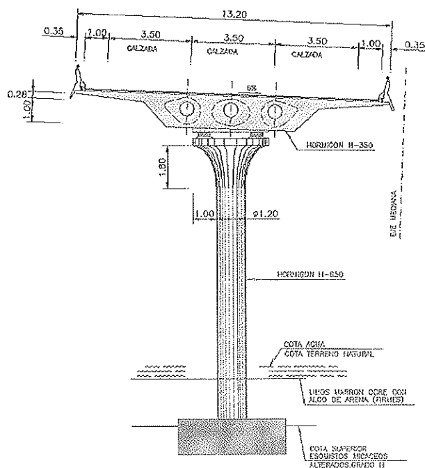
Figura 3. Dovelas de pila.
