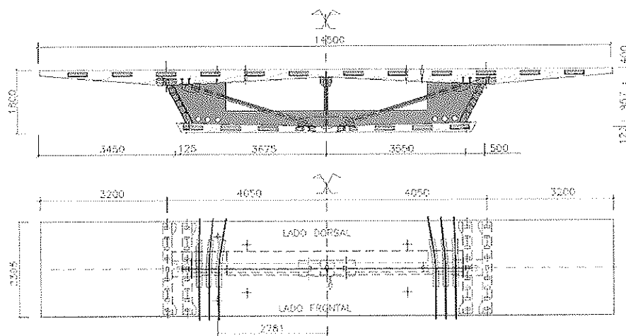
Figura 9. Dovela con desviadores de los tendones de pretensado.
