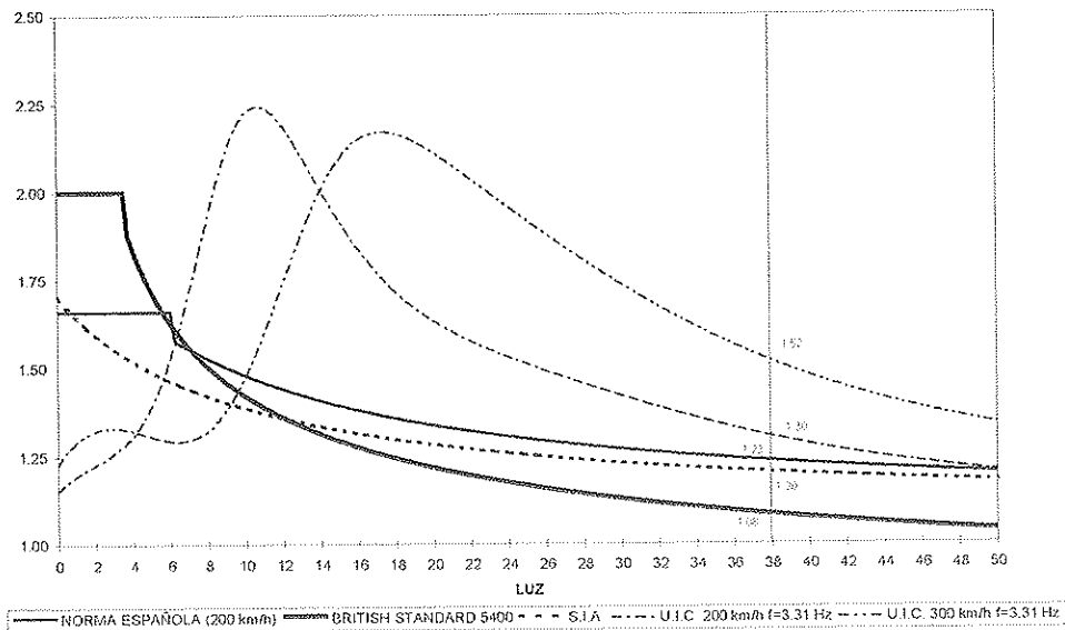
Figura N.º 9. Coeficiente de impacto según distintas normativas europeas.
