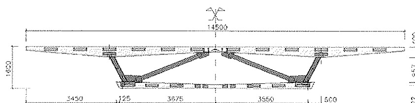
Figura 4. Dovela con cuaderna tipo A.
