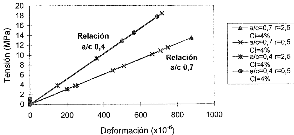
Figura 5. Comportamiento tensión-deformación del recubrimiento de hormigón, con la evolución de la corrosión de la armadura, para los hormigones con 4% de CaCl 2 .
