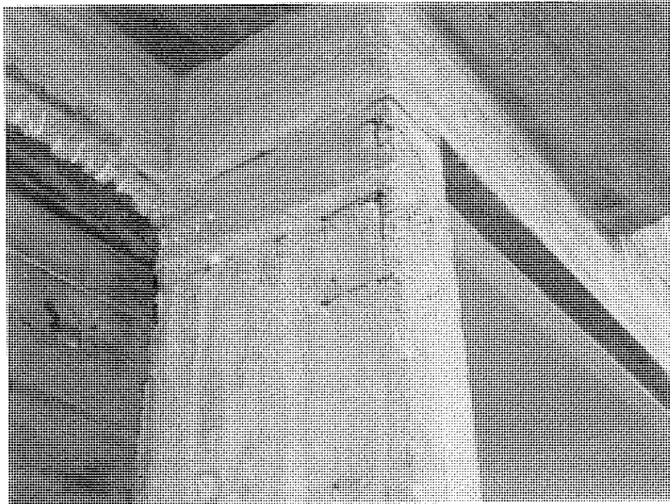
Foto 11. Estructura en construcción donde se detecta la falta de recubrimiento.
