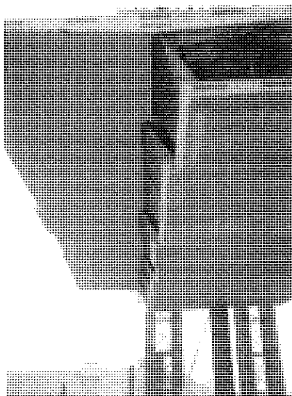
Figura 20. Cuelgue de dovelas previo al ajuste geométrico
