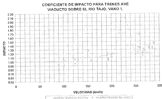
Figura N.º 7. Coeficiente de impacto en vano 1.
