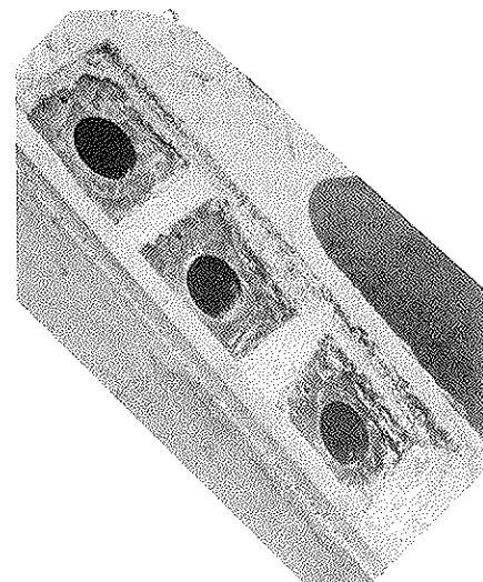
Figura 4. Detalle de placa de anclaje en las almas
