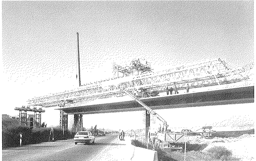
Figura 21. Autolanzamiento de cimbra.
