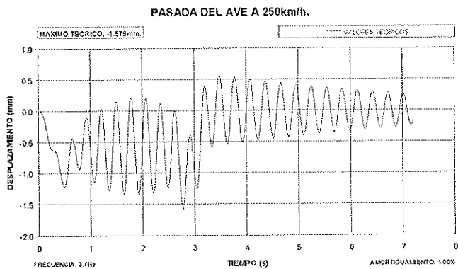
Figura N.º 11 (Cont.). Comportamiento teórico para distintas velocidades del tren de cargas.
