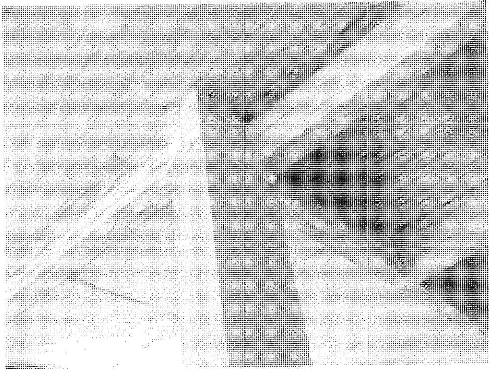
Foto 14. Vigas excéntricas llegando a un pilar y deficiencias de configuración.
