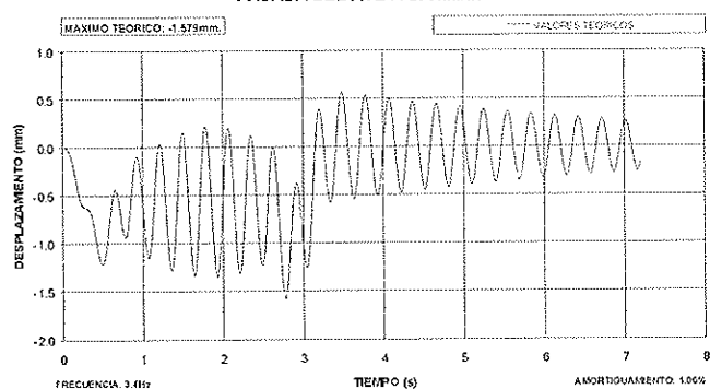
Figura N.º 11 (Cont.). Comportamiento teórico para distintas velocidades del tren de cargas.
