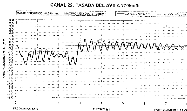
Figura N.º 5. Prueba Dinámica 05.
