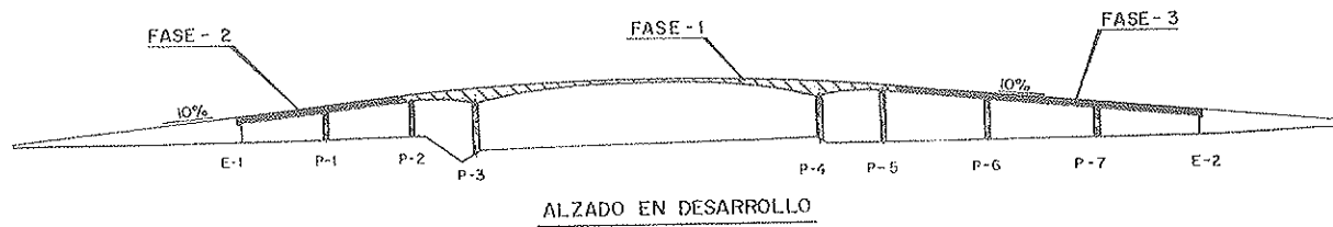
Figura 8. Fases de construcción del tablero.
