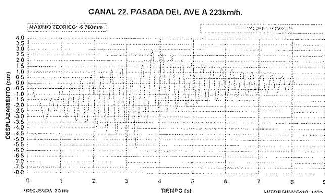
Figura N.º 17. Composiciones AVE. Modelo teórico para la velocidad crítica.
