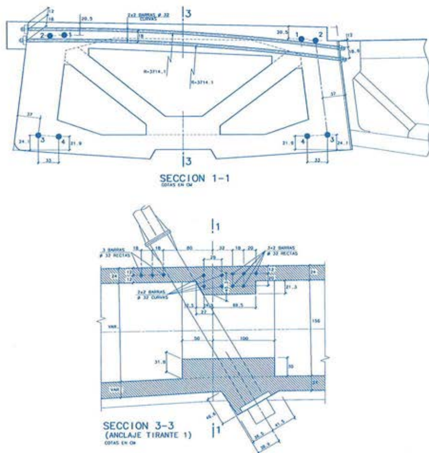
Figura 11: Detalles del diedro de anclaje de un tirante.
