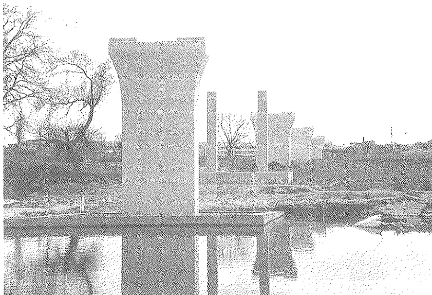
Figura 8. Vista general de pilas, con el apeo de montaje en el vano adyacente al río.
