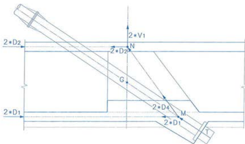
Figura 12: Esquema de las bielas de fuerzas en un anclaje de tirante vistas en Alzado (2D).
