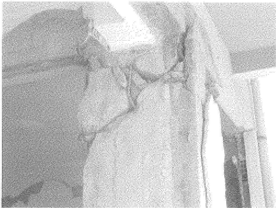
Foto 10. Fallo de pilar donde se puede apreciar poco acero de refuerzo.
