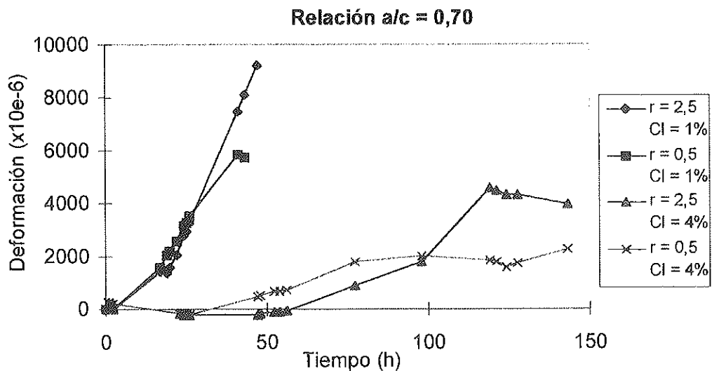
Figura 3. Evolución de las deformaciones en el tiempo para las familias de hormigones con relación a/c = 0,70 .
