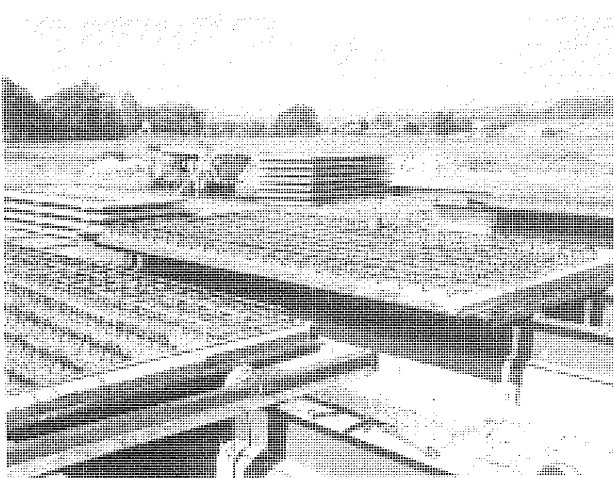
Figura 6. Fabricación y acopio de placas prefabricadas para la losa superior.
