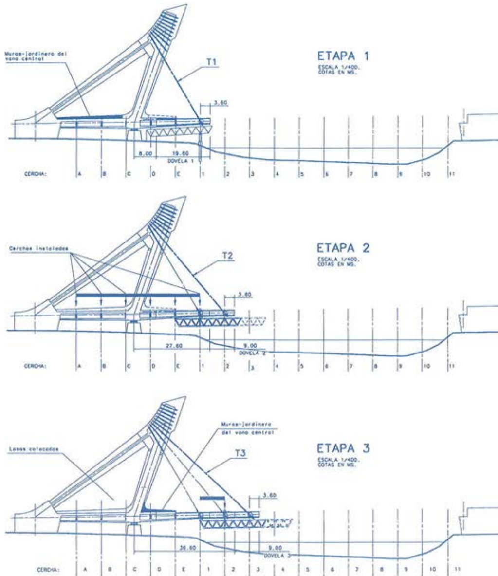
AVANCE EN VOLADIZO: ETAPAS 1 A 3
