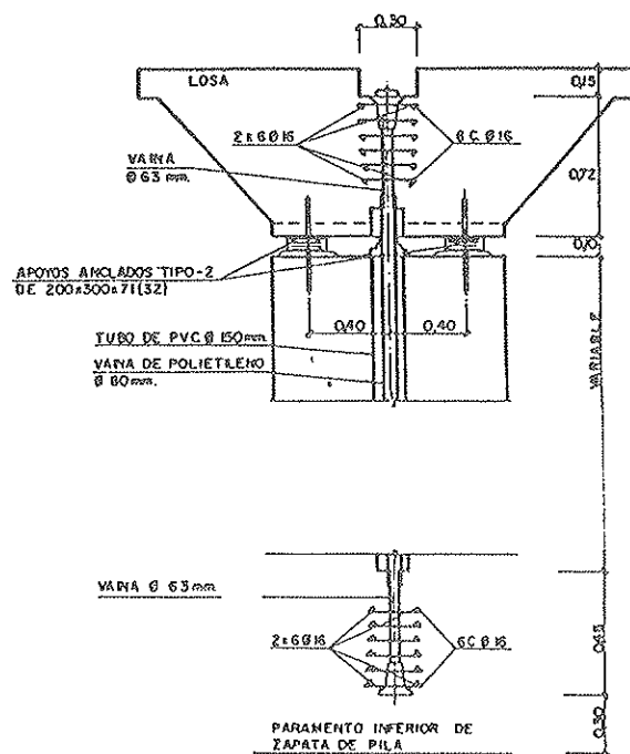
Figura 7. Pretensado vertical en pilas 2 y 5.
