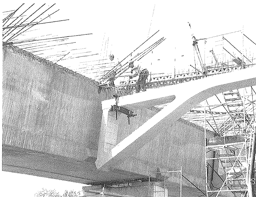
Figura 5. Pieza prefabricada de voladizo en montaje.
