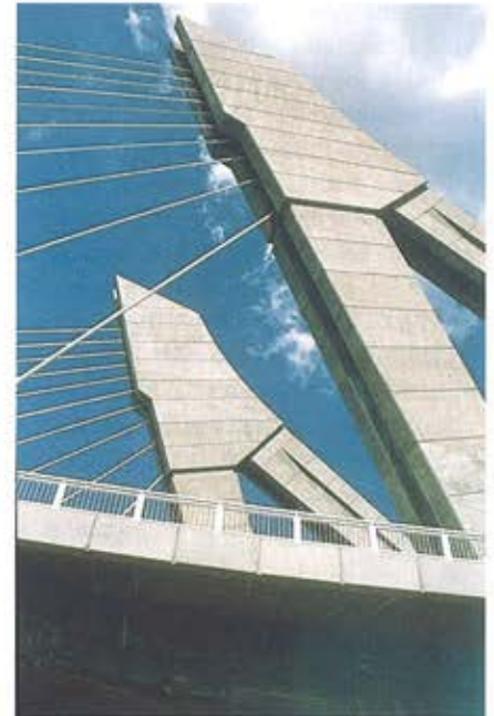
Figura 14. Mástiles y cabezas de anclaje marcan los dos planos de suspensión del tablero. Figure 14. Pylons and heads indicate the vertical planes of suspension of the deck.
