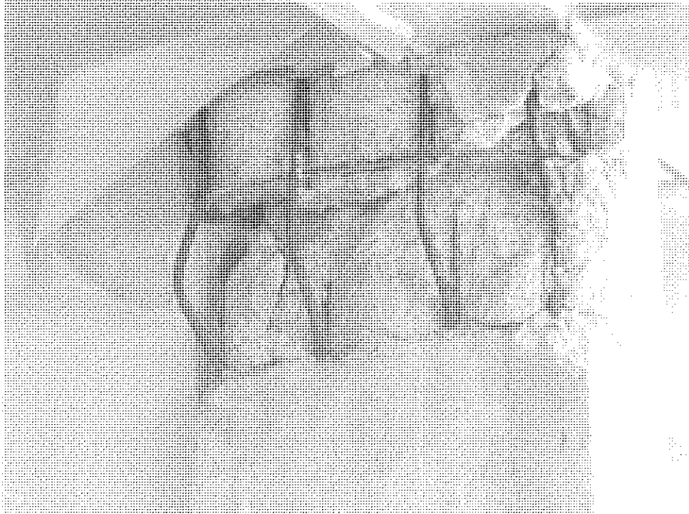
Foto 9. Pilar fallado con poco acero trasversal y alta corrosión.
