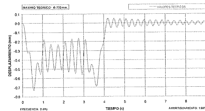
Figura N.º 12. Comportamiento teórico para distintos valores de la rigidez del tablero (con f = \text{constante} ).
