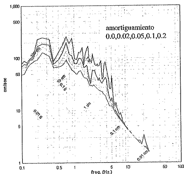
Figura 4. Espectro de respuesta para el registro de aceleración en Yarımcı.
