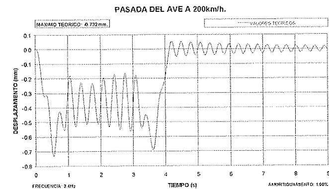
Figura N.º 12. Comportamiento teórico para distintos valores de la rigidez del tablero (con f = \text{constante} ).
