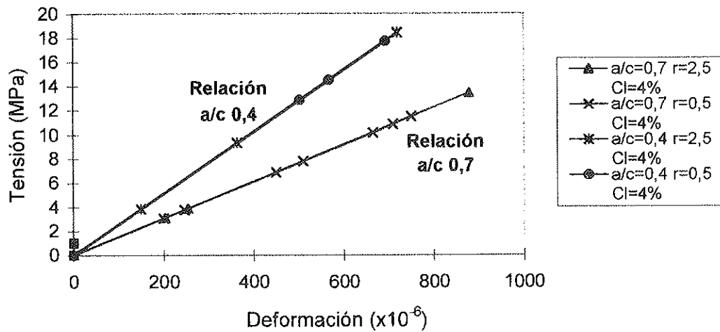
Figura 5. Comportamiento tensión-deformación del recubrimiento de hormigón, con la evolución de la corrosión de la armadura, para los hormigones con 4% de CaCl 2 .
