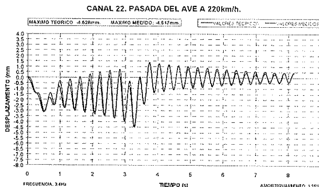
Figura N.º 3. Prueba Dinámica 06.
