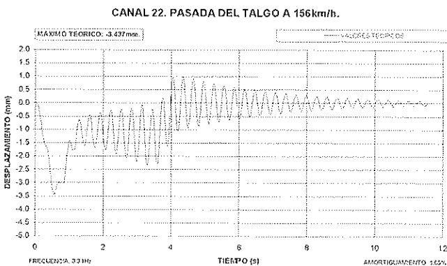
Figura N.º 16. Composiciones TALGO. Modelo teórico para la velocidad crítica.
