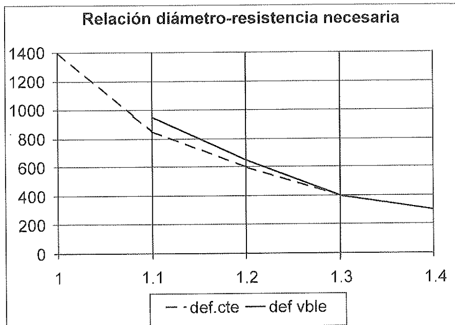
Figura 13. Relación diámetro-resistencia necesaria.
