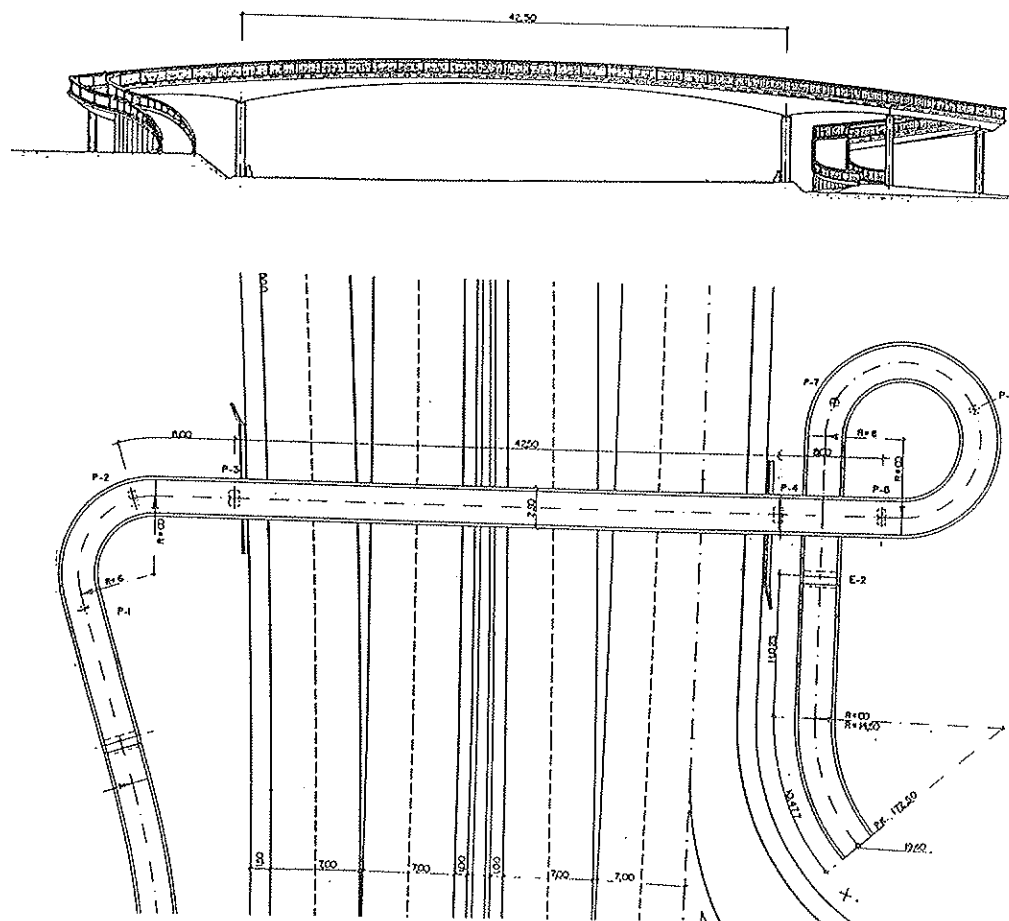
Figura 2. Pasarela. Alzado y Planta general.
