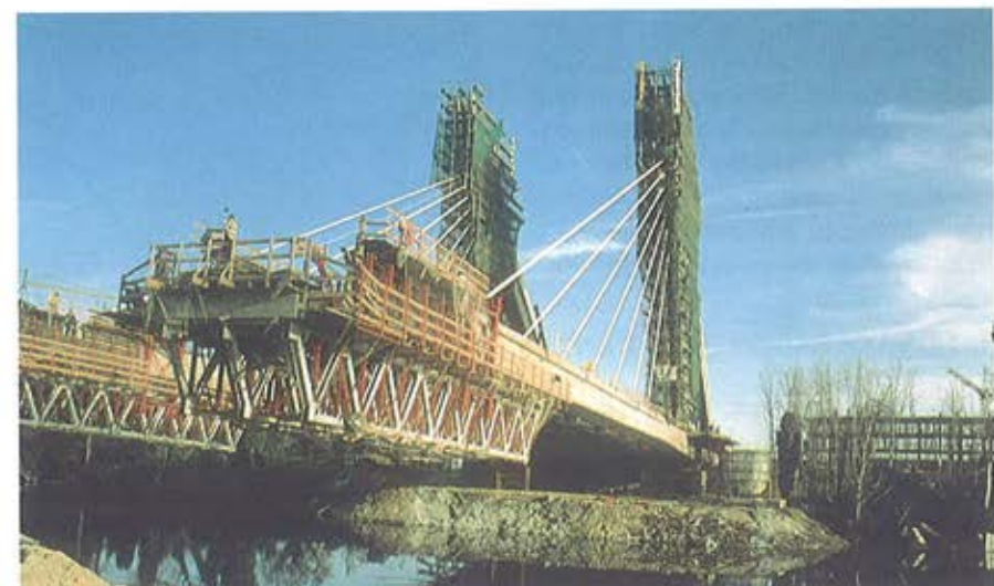
Foto 7. Carros de avance vistos desde la margen derecha.
