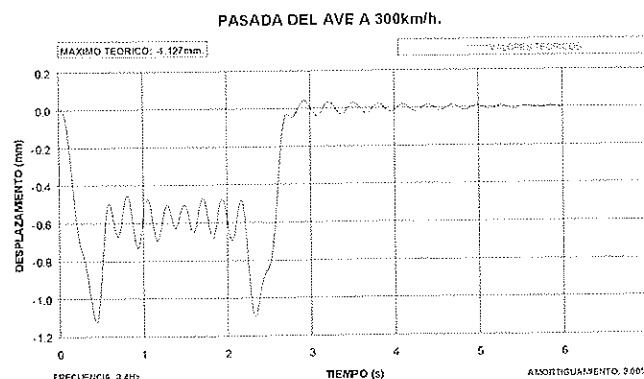
Figura N.º 14 (Cont.). Comportamiento teórico para distintos valores del amortiguamiento del tablero. Puede apreciarse que la velocidad crítica no varía.
