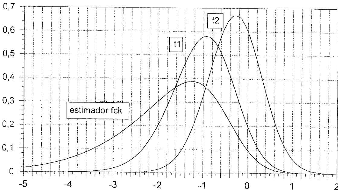
Figura 1. Funciones de densidad de probabilidad del estimador tipificado con cuatro determinaciones y sus componentes.
