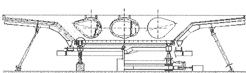
Figura 7. Molde de dovelas.
