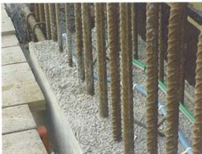
Figura 6.5.7. Junta de hormigonado.
