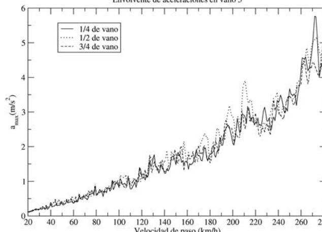
Figura 24. Envoltorio de aceleraciones en puntos del vano 5
