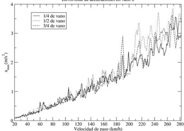
Figura 21. Envolvente de aceleraciones en puntos del vano 2
