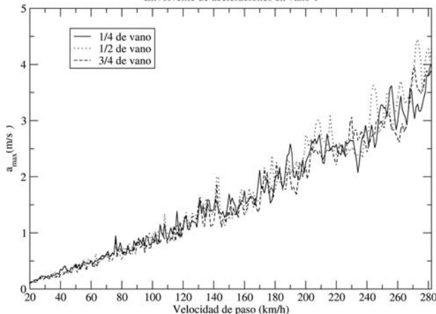
Figura 20. Envolvente de aceleraciones en puntos del vano 1
