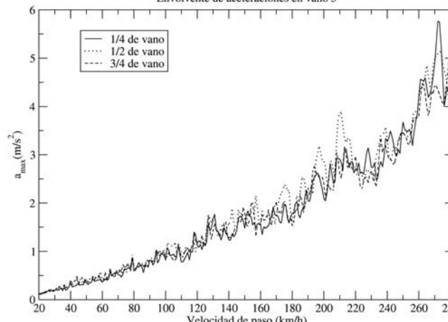
Figura 24. Envolvente de aceleraciones en puntos del vano 5
