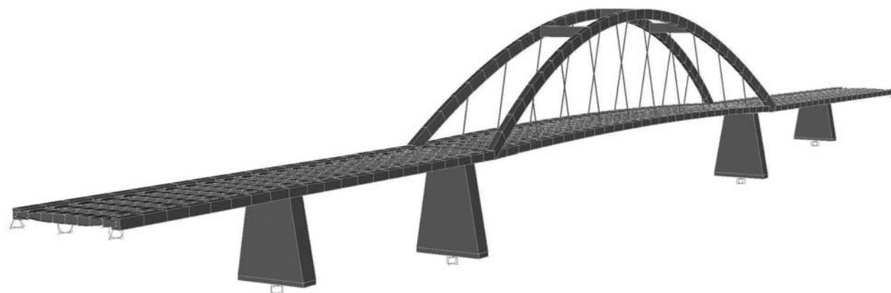
Figura 10. Modelo inicial con placas y vigas sin colaboración de losa. En éste se incluían también las pilas
