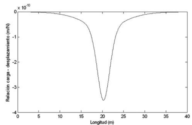
Figura 16. Relación carga-desplazamiento
