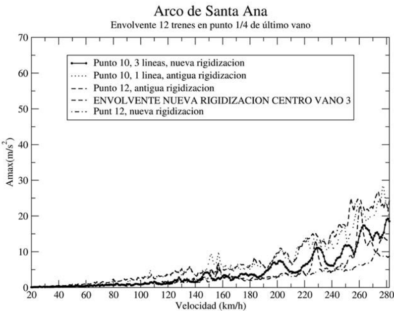
Figura 12. Comparativa de aceleraciones respecto a modelo previo
