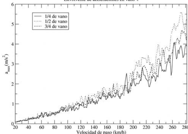
Figura 23. Envolvente de aceleraciones en puntos del vano 4
