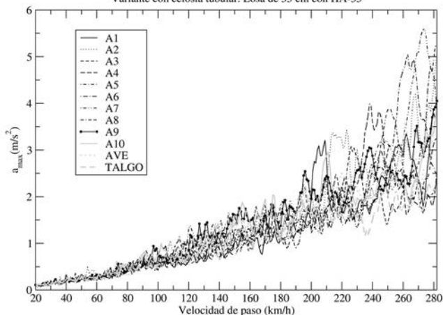
Figura 19. Envolvente de aceleraciones. Composición por trenes
