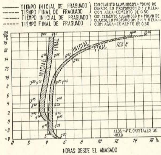
Fig. 10.—Tiempos de fraguado de morteros con cemento Portland. Fig. 11.—Tiempos de fraguado con morteros de cemento aluminoso. Fig. 12.—Ensayo de congelación de probetas de siete días, guardadas en posición horizontal. Fig. 13.—Ensayo de congelación con probetas de doce horas de edad, conservadas en posición horizontal. En 8 de las 9 probetas, los tapones fueron expulsados de los tubos, y, en una de ellas, el tubo se rompió. Fig. 14.—Comparación de viscosidades de morteros amasados con dos cementos aluminosos L y R, y polvo de cuarzo en la proporción 2:1, con diferentes relaciones de agua-cemento.
